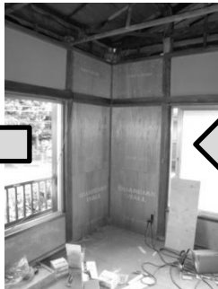
補強壁設置
