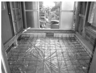
基礎補強中
